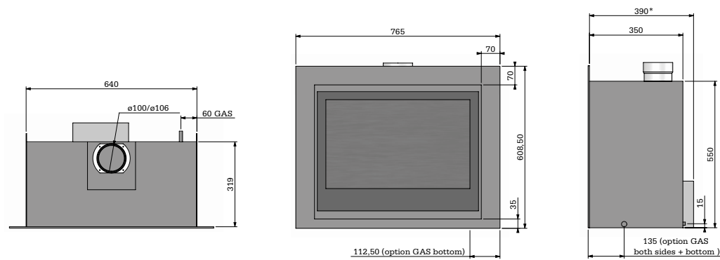
Unica-2 70 - 4 sided frame 70 mm * Standard depth: 350 mm. Including optional fan system: 390 mm. Profondeur standard : 350 mm et set de ventilation optionnel inclus : 390 mm
