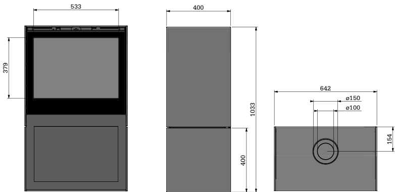
BOX gas 55 - met opslagmodule, with storage module, avec socle, con modulo rialzo
