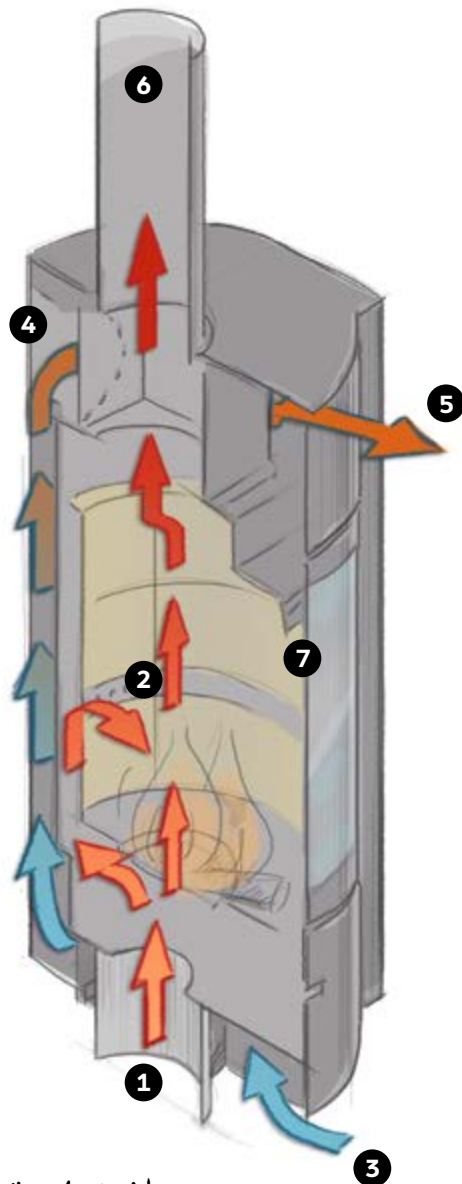
Verbrandingstechniek en luchtcirculatie Stuv 30
