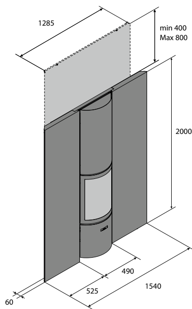
Stûv 30-in hoekbekleding
