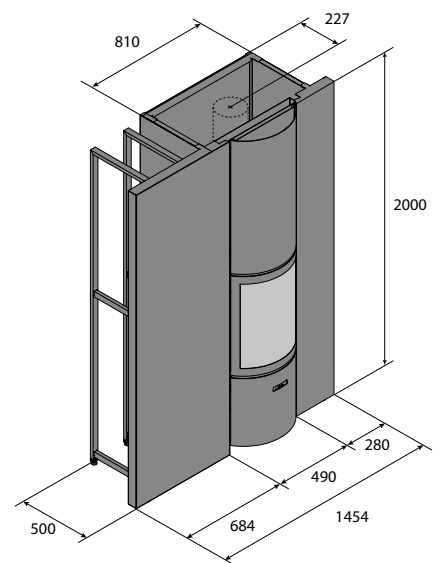
Stûv 30-in plaatsklare schouw
